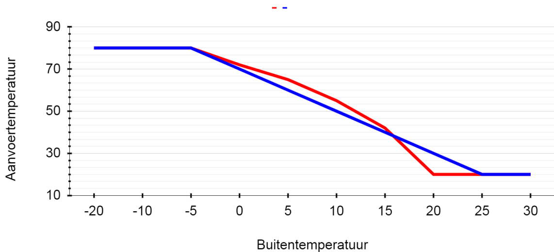
Stooklijn radiatorgroep
